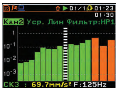
1/3 октавный спектр в диапазоне центральных частот от 0,4 Гц до 2,5 кГц
